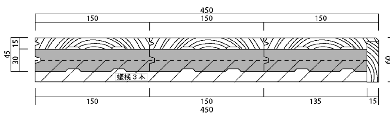
圧密式台 加工形状
